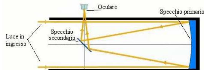
Schema di un telescopio riflettore
